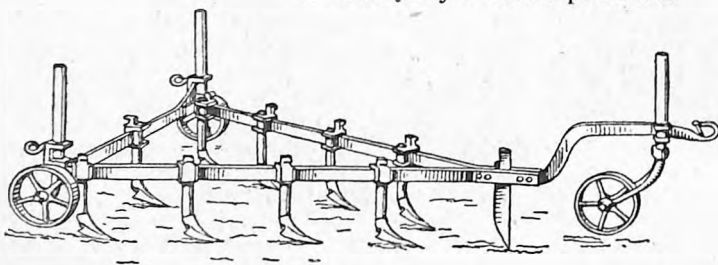
5. Spulchniacz.
