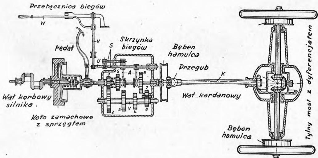
2. Przeniesienie siły (schemat).
