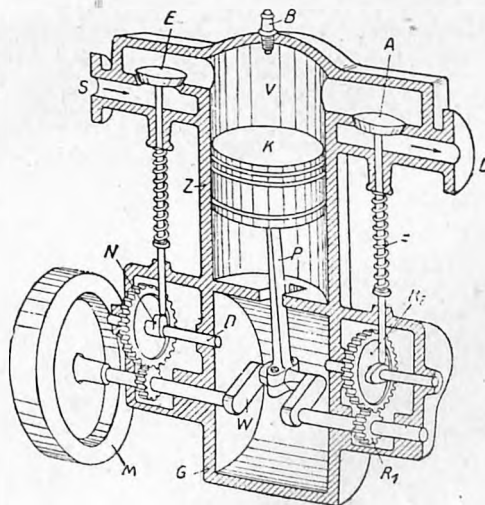
6. Silnik spalinowy (schemat).
