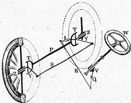
5. Schemat mechanizmu kierowniczego.
