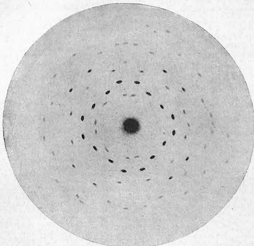
1. Röntgenogram blendy cynkowej (wiązka prostopadła do płaszczyzny sześciianu).
