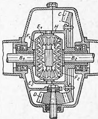
4. Przekrój dyferencjału.
