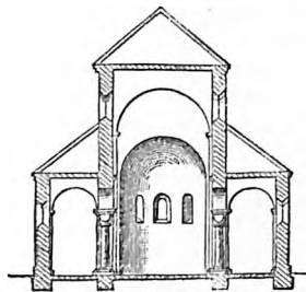
Przekrój poprzeczny bazyliki romańskiej.
