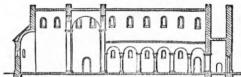
Przekrój podłużny bazyliki romańskiej.
