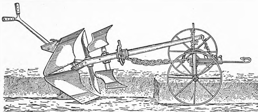
1. Pług przekładny (bliźniaczy).
