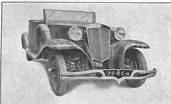
Samochód z napędem na przednie koła i niezależnym resorowaniem.
