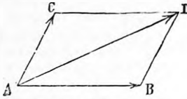
Równoległobok sił.
