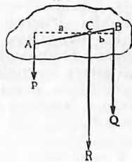
Równoległe siły.
