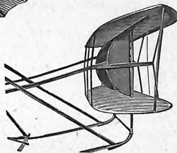
6. Stery samolotu Wrighta.
