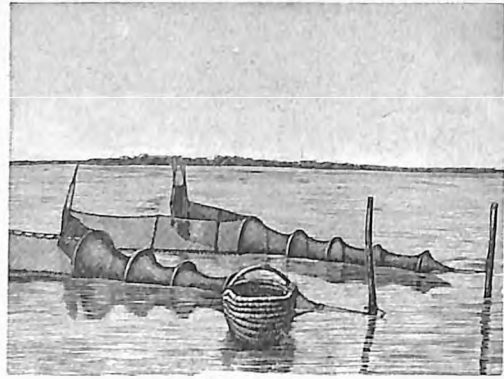
2. Żaki węgorskie.
