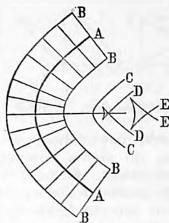
Równoległe krzywe.
