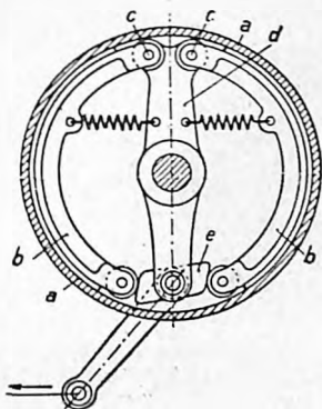
3. Hamulec szczękowy (wewnętrzny).
