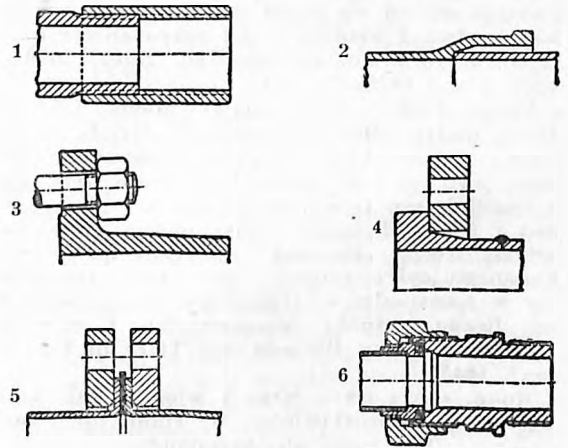
Polączenia rurowe.
